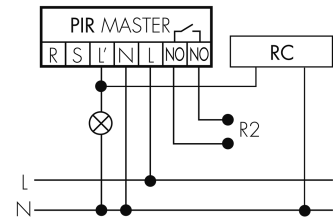
Fonctionnement normal avec circuit RC
