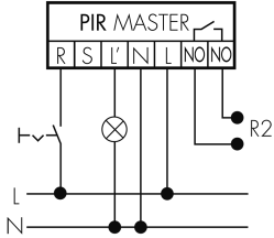
Fonctionnement Master-Slave
