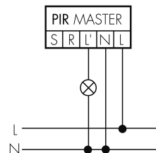
Funzione ad impulso sulla minuteria
