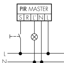
Funzione con commutatore rotativo «Manuale - 0 - Automatico»
