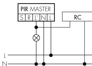
Funzionamento normale con filtro RC
