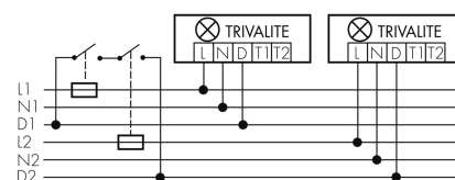
Funzionamento gruppi/Funzionamento sistema attraverso 2 gruppi fusibili
