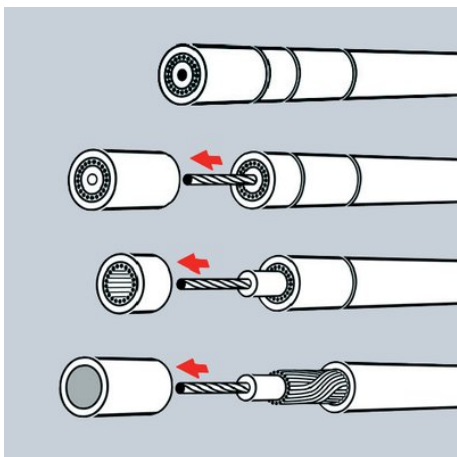
Dreistufige Abisolierung eines Koaxialkabels
