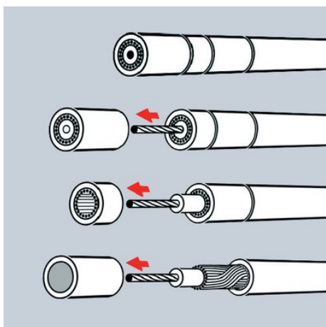
Dénudage en trois étapes d'un câble coaxial
